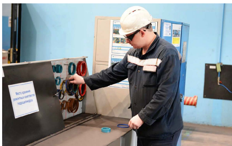
▲ Организация рабочего места на участке по ремонту гидроцилиндров
